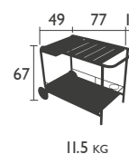
4164 - BEISTELLTISCH / ROLLENDE BAR Abnehmbare Tischplatte aus Aluminium Struktur aus Aluminiumrohr Tischplatte aus Aluminiumblech
